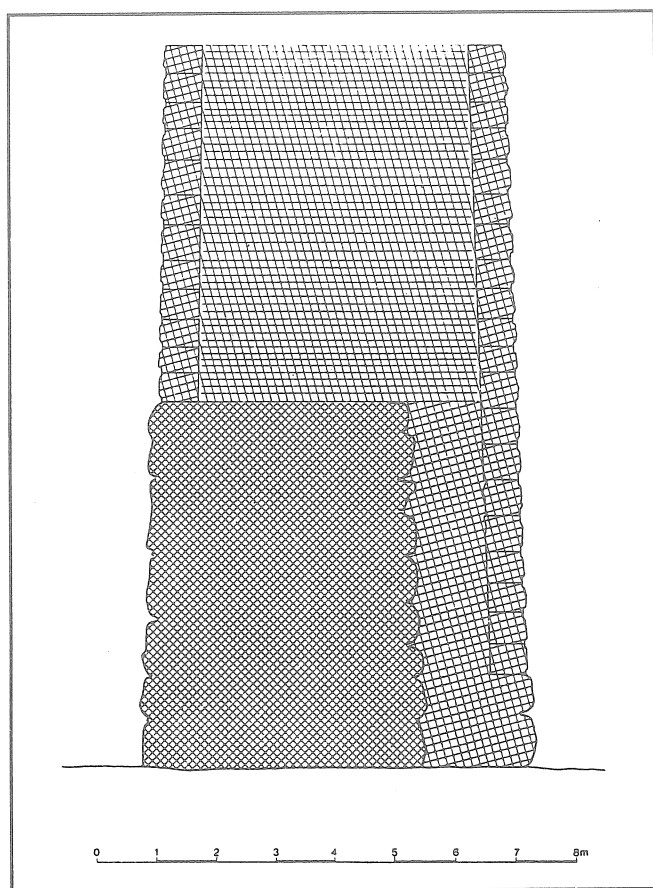
Fig. 2. - Superposició dels dos llenços murals, segons Hauschild (1979).
