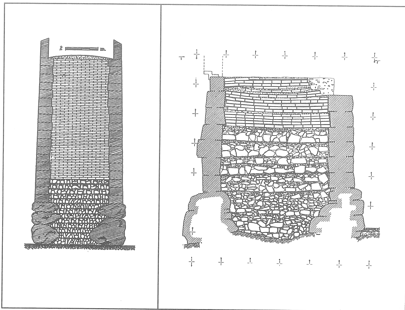
Fig. 1 a. - Secció teòrica de l'estructura de la muralla (segona fase), segons Serra Vilaró (1949).
