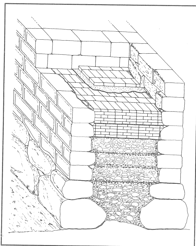
Fig. 15. - Restitució de la part baixa de la muralla, il·lustrativa de la tècnica constructiva utilitzada.
