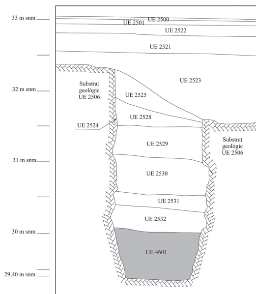
Figura 3. Secció del pou UE 2524. He destacat en color gris la UE 4601, objecte d'aquesta notícia. Escala 1:50.
