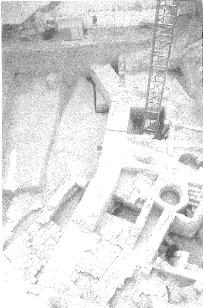
Foto núm 1. Vista aèria on s'aprecien els fonaments de les dues torres, la muralla cristiana i les construccions de l'interior de la ciutat.
