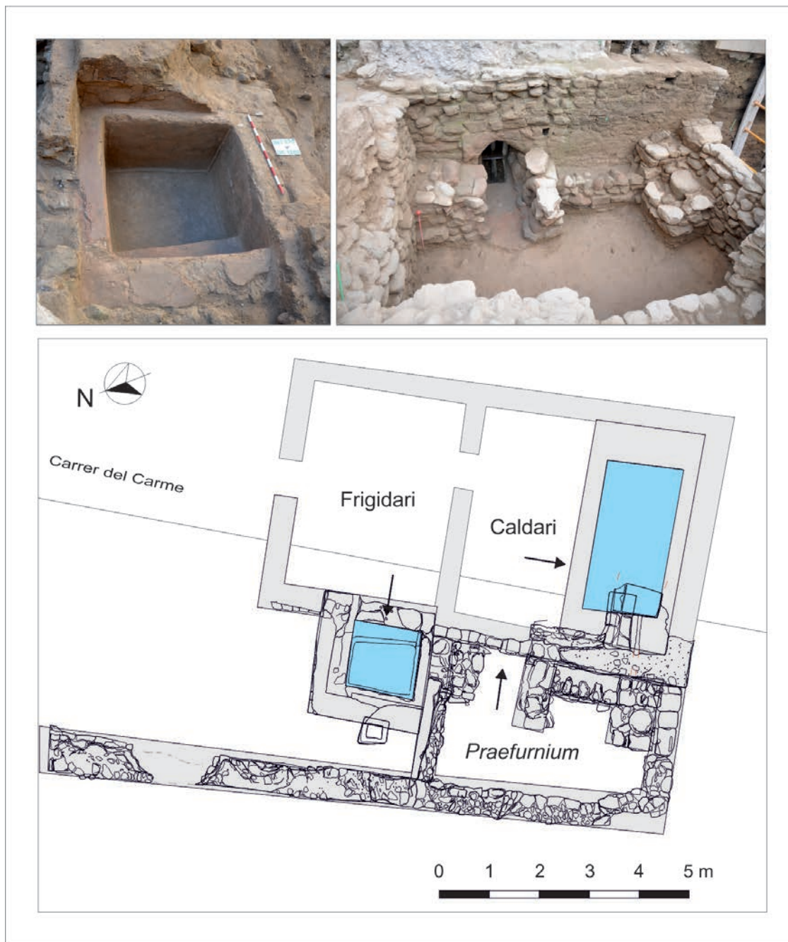
Figura 9. Int 270. Carrer del Carme, 9-11. Planta i restitució d'unes termes domèstiques.
