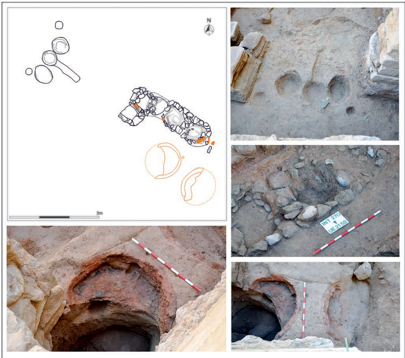
Figura 10. Int 270. Planta i detalls dels retalls practicats a l'argila pertanyents a possibles forns de fusió.
