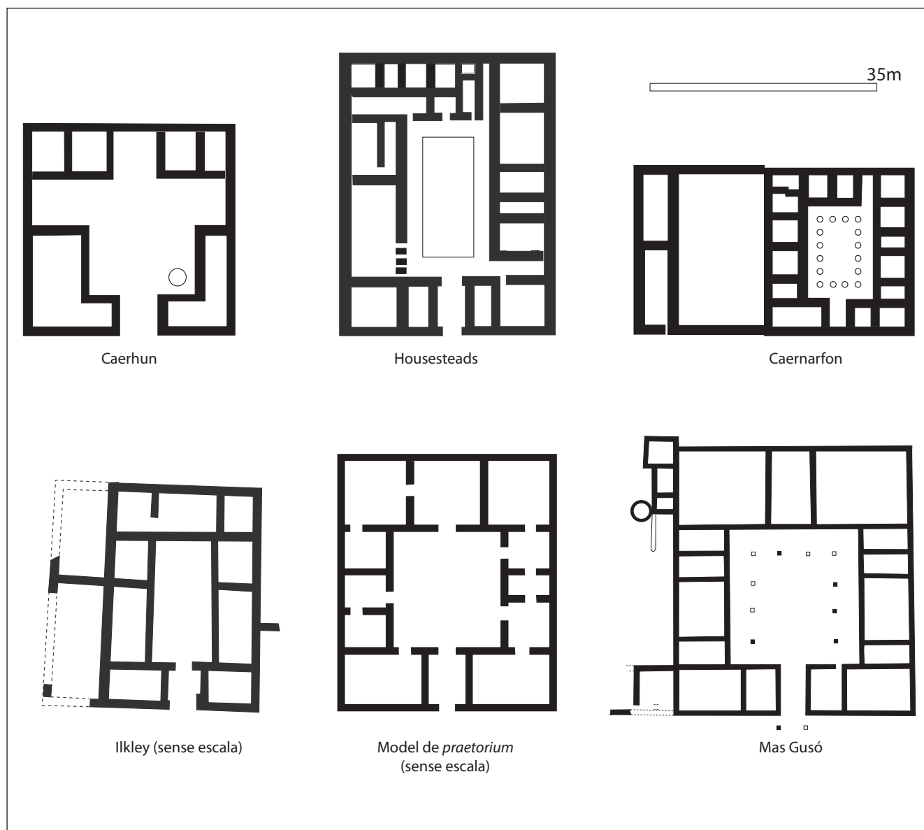
Figura 7. Plantes comparatives amb estructures similars de Caerhun, Housesteads, Caernarfon, Ilkley (a partir de Wilson 1980) i Mas Gusó.
