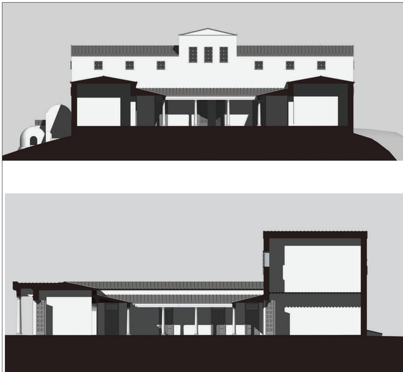
10. Mas Gusó. Proposta idealitzada de restitució de la statio a la fase 3. A dalt, secció est-oest. A baix, secció nord-sud.
