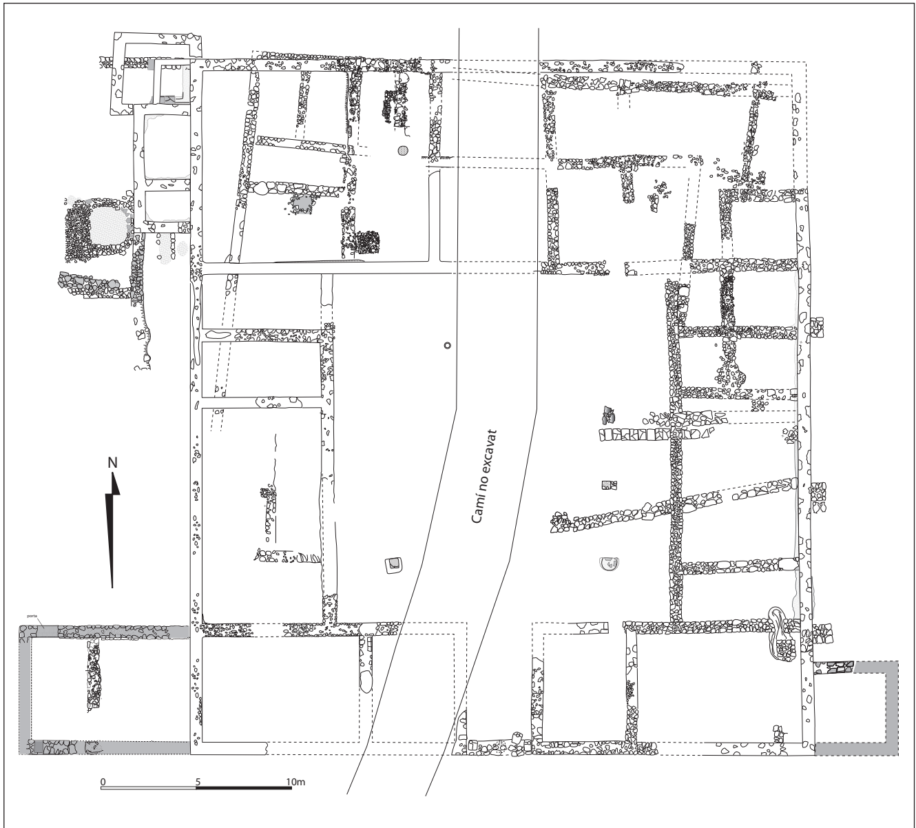
Figura 2. Mas Gusó. Planta general amb totes les estructures d'època romana.
