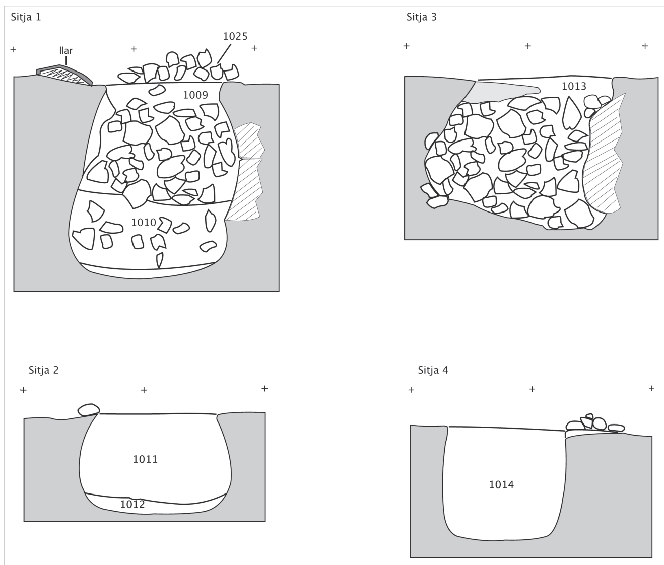
Fig. 8. Seccions estratigràfiques de les quatre primeres sitges.
