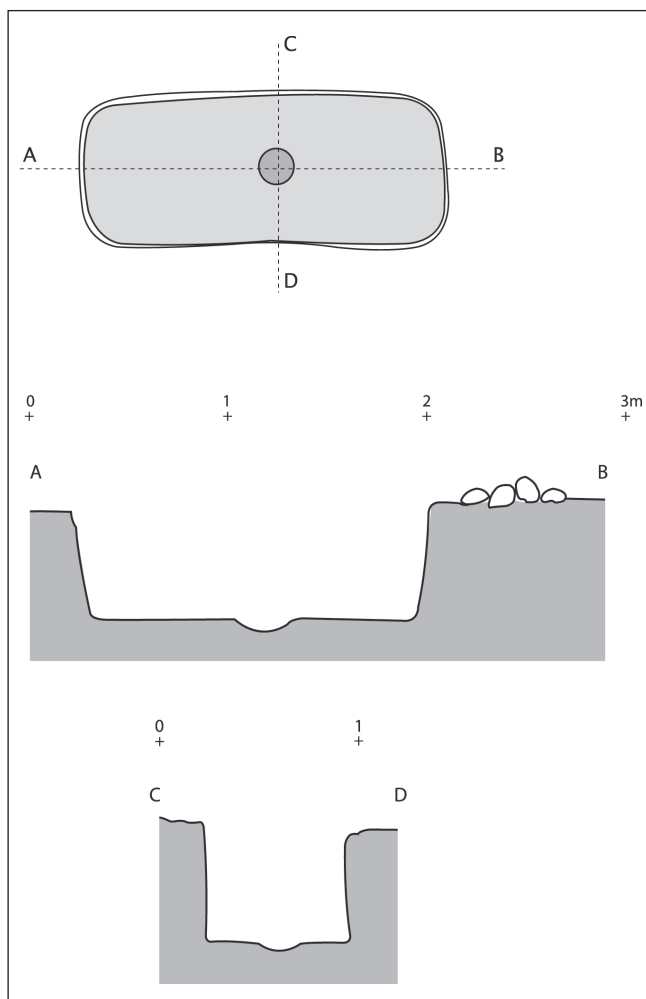
Fig. 6. Planta i seccions del dipòsit per a líquids.
