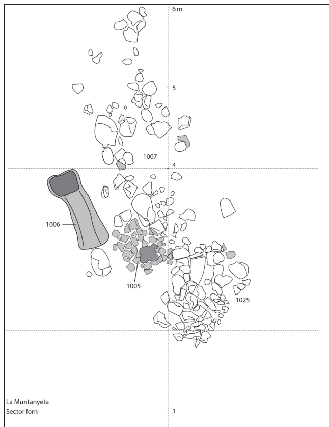
Fig. 4. Planta de l'espai de ponent, amb una llar domèstica (1005) i un forn per a metalls (1006).
