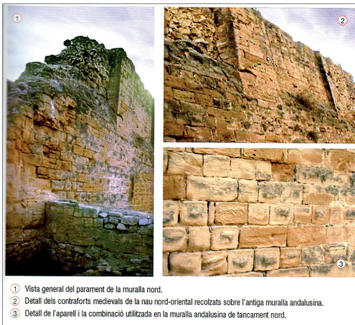
Figura 14. Tipus de parament utilitzat en el tancament nord de la Suda de Lleida (foto: Secció d'Arqueologia de l'Ajuntament de Lleida, a Gil et al. 2007: 51, figura 14).
