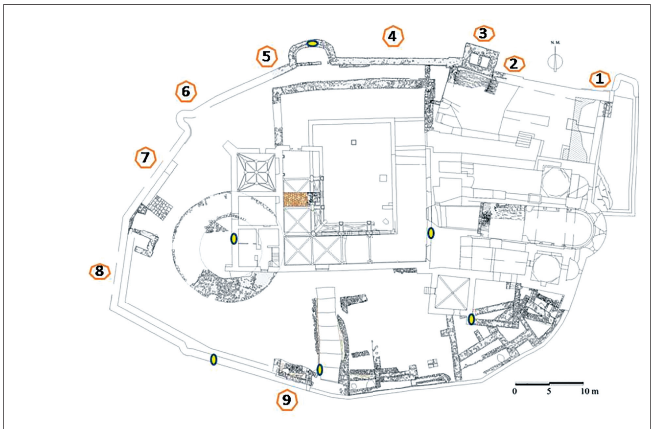
Figura 5. Plànol del recinte fortificat de Sant Pere d'Àger amb enumeració dels sectors. Planta del recinte proporcionada per Josep M. Vila. Publicada a Maragall i Vila 2005. Els cercles grocs indiquen indrets on s'han identificat carreus reutilitzats.
