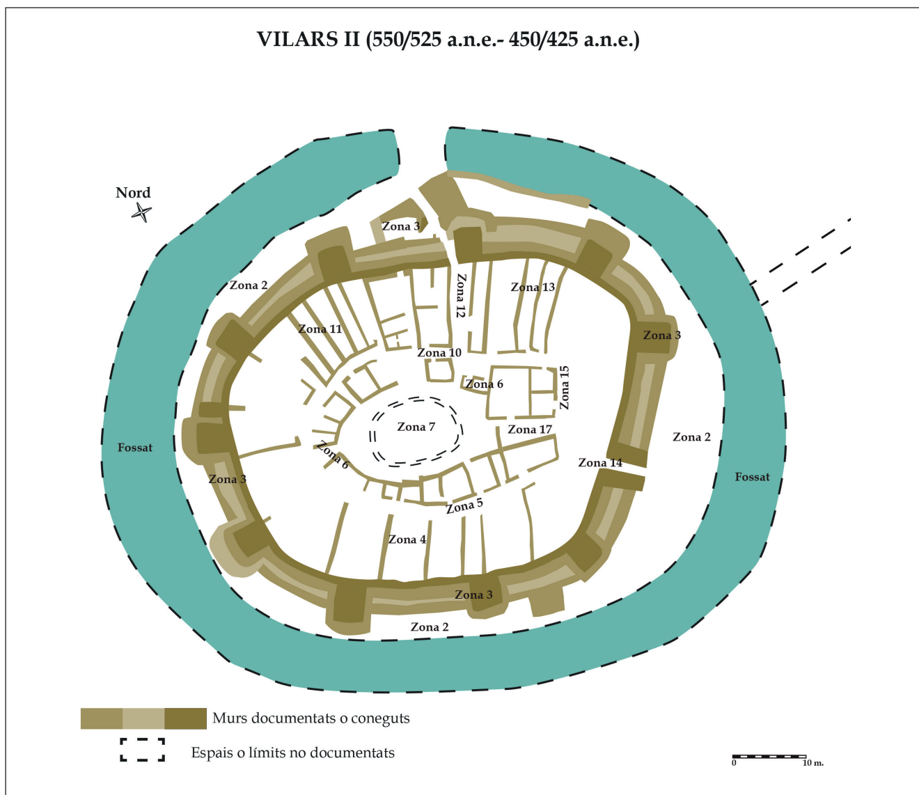
Figura 5. Planta general amb totes les zones on es documenta la fase Vilars II (550-450 ane). Font: GIP 2016.
