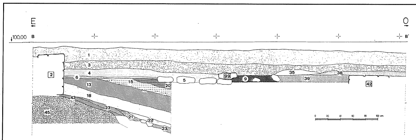
Figura 9. - Secció est-oest a la zona central.
