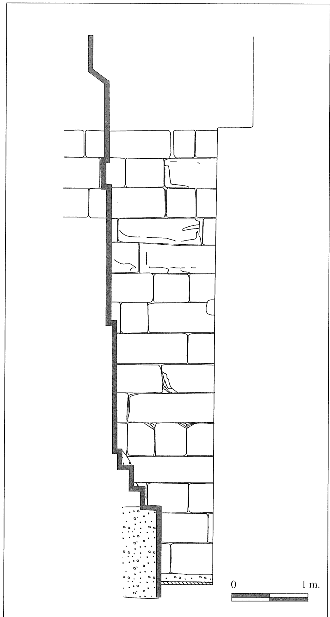
Fig. 3. Alçat del mur andalusí documentat a la cala 4 realitzada a l'interior de la Seu Vella (Int-70). Segons el dibuix de M. Cargol i J. M. Sabaté (Pla Director de la Seu Vella, 1993).
