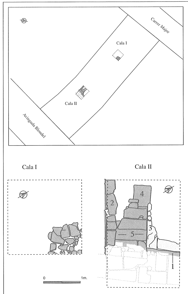
Fig. 10. Estructures andalusines (segles XI) documentades al carrer Major núm. 17 (Int-13) segons els plànols de L. Sant (GARCÉS i GALLART, 1986).
